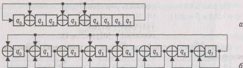
Рис. 3.19. Поле GF(2^8) :
